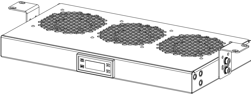
Модуль вентиляторный R-FAN-6K-1U Вариант установки-1 Масса = 7 кг
