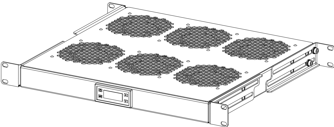
Модуль вентиляторный R-FAN-6K-1U Вариант установки-1 Масса = 7 кг
