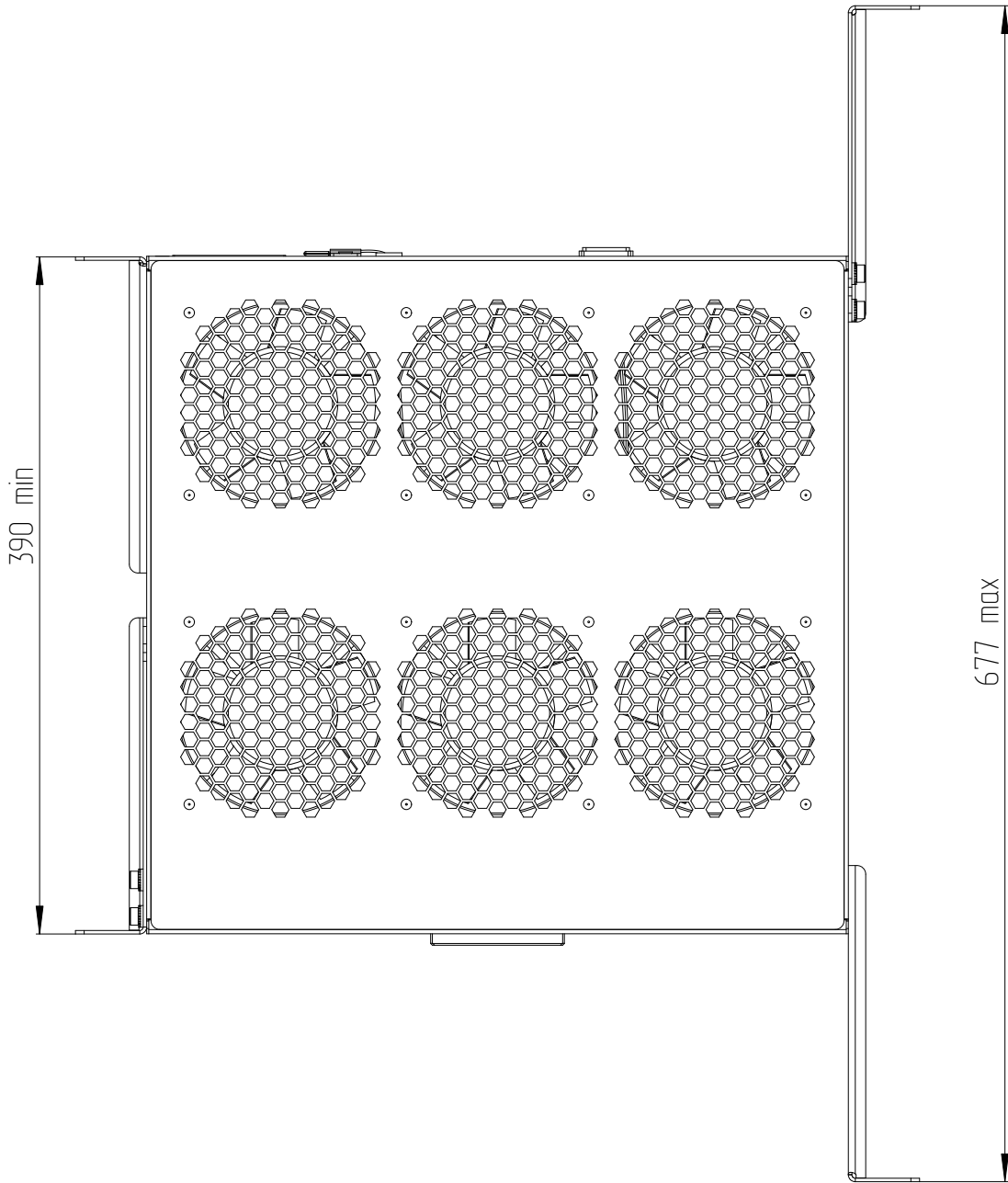
R-FAN-6K-1U Глубина Установки в шкаф
