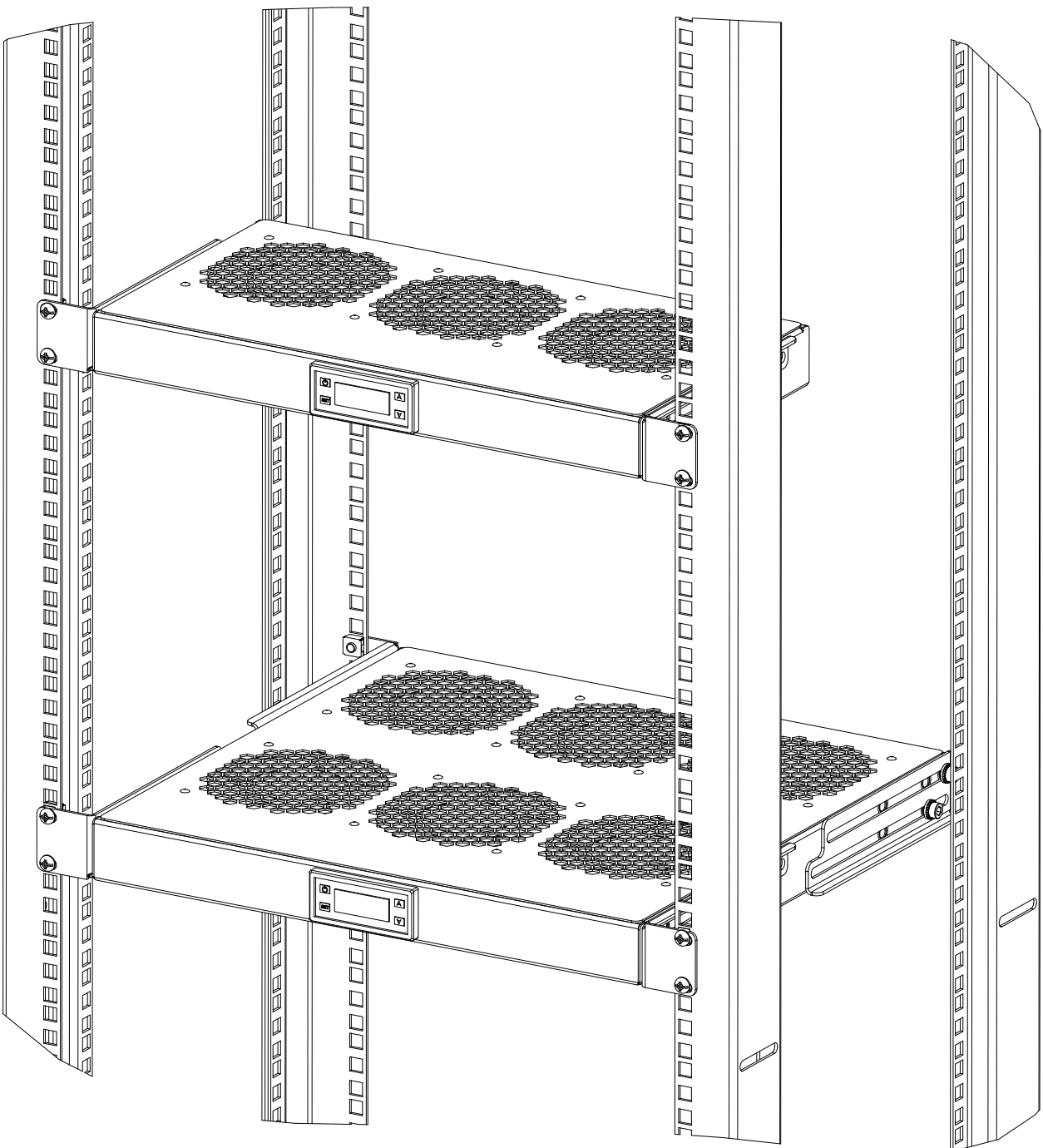
Установка изделия R-FAN-3K-1U R-FAN-6K-1U в юнитовые направляющие
