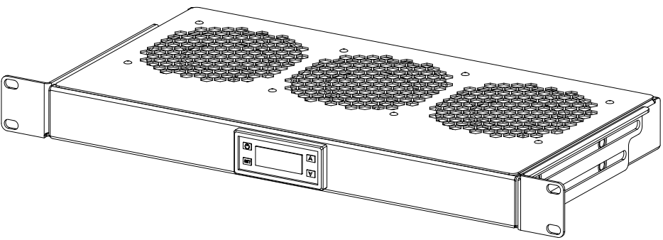
Модуль вентиляторный R-FAN-3K-1U Вариант установки-2
