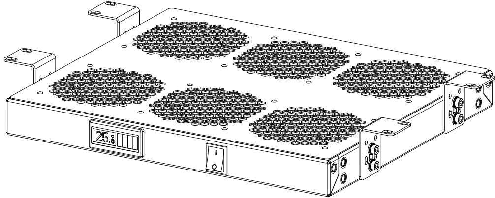
Модуль вентиляторный R-FAN-6-1U Вариант установки-2
