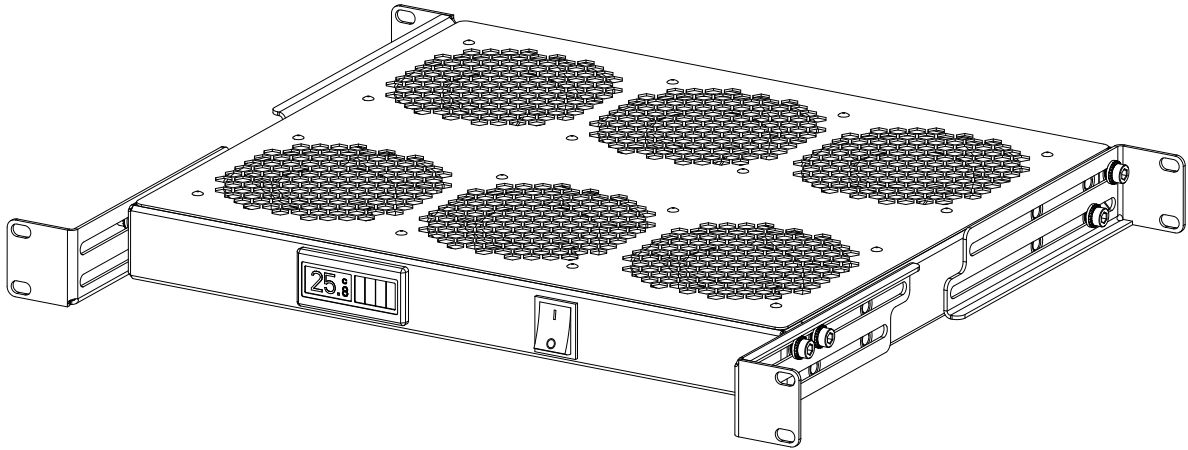
Модуль вентиляторный R-FAN-6-1U Вариант установки-2
