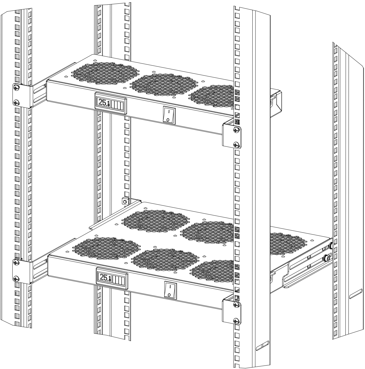
Установка изделия R-FAN-3-1U R-FAN-6-1U в юнитовые направляющие
