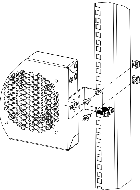
Схема крепления в вертикальном положении R-FAN-3-1U R-FAN-3K-1U К юнитовым направляющим
