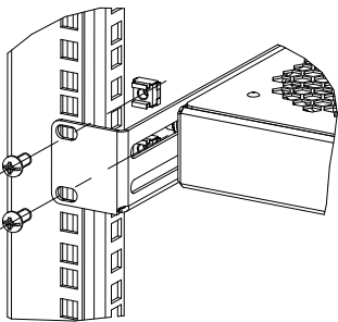
Схема крепления R-FAN-3-1U R-FAN-6-1U R-FAN-3K-1U R-FAN-6K-1U К юнитовым направляющим
