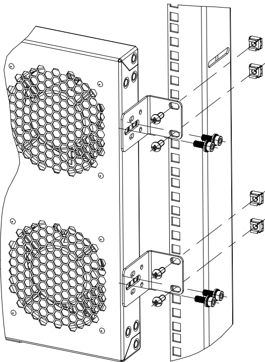
Схема крепления в вертикальном положении R-FAN-6-1U R-FAN-6K-1U К юнитовым направляющим
